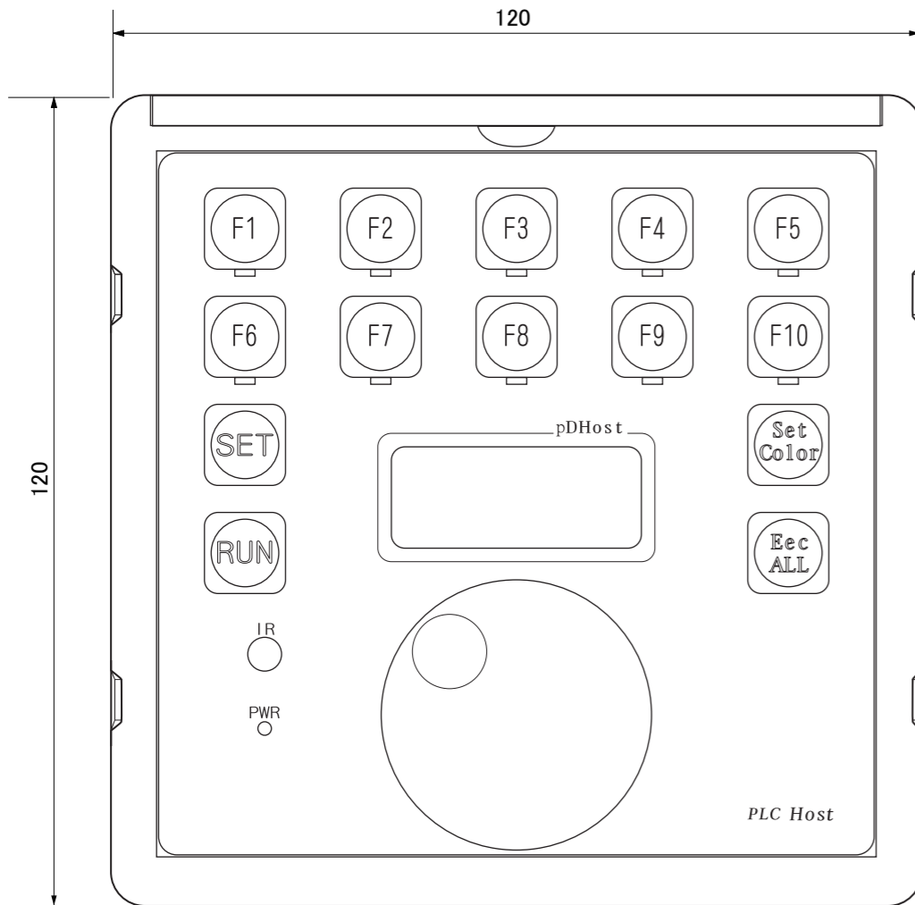
【正面図】
