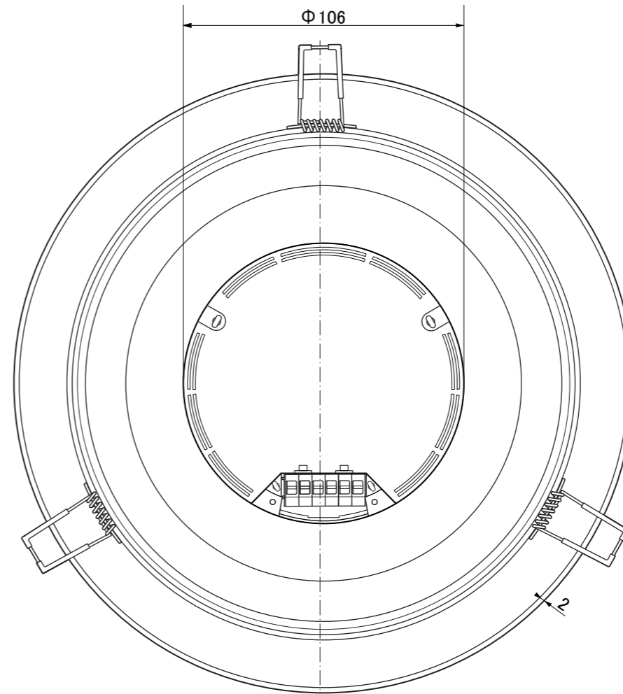
【底面図】
