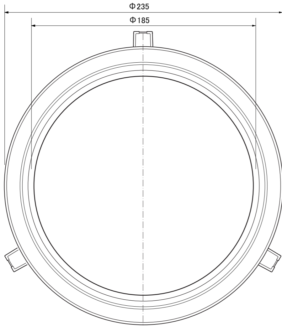
【上面図】
