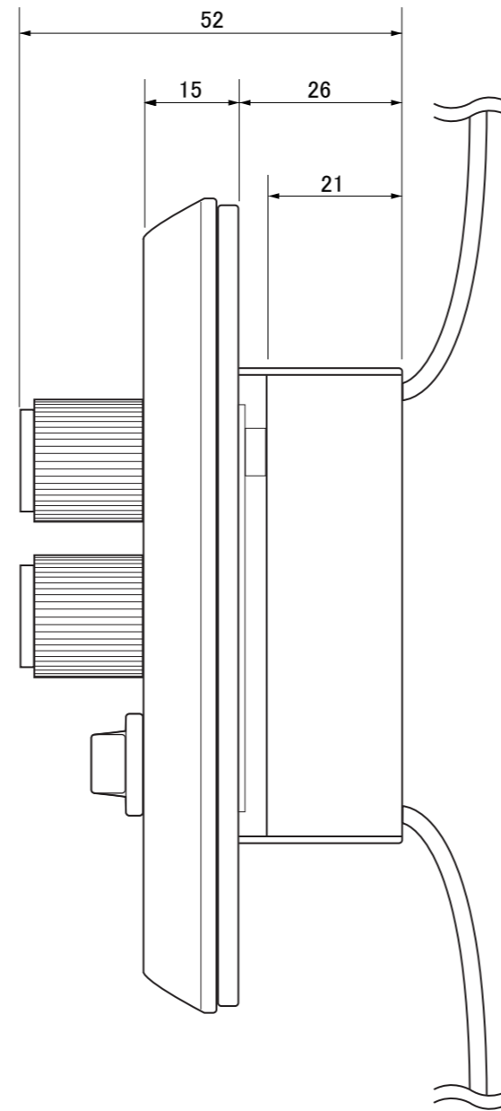
【側面図】
