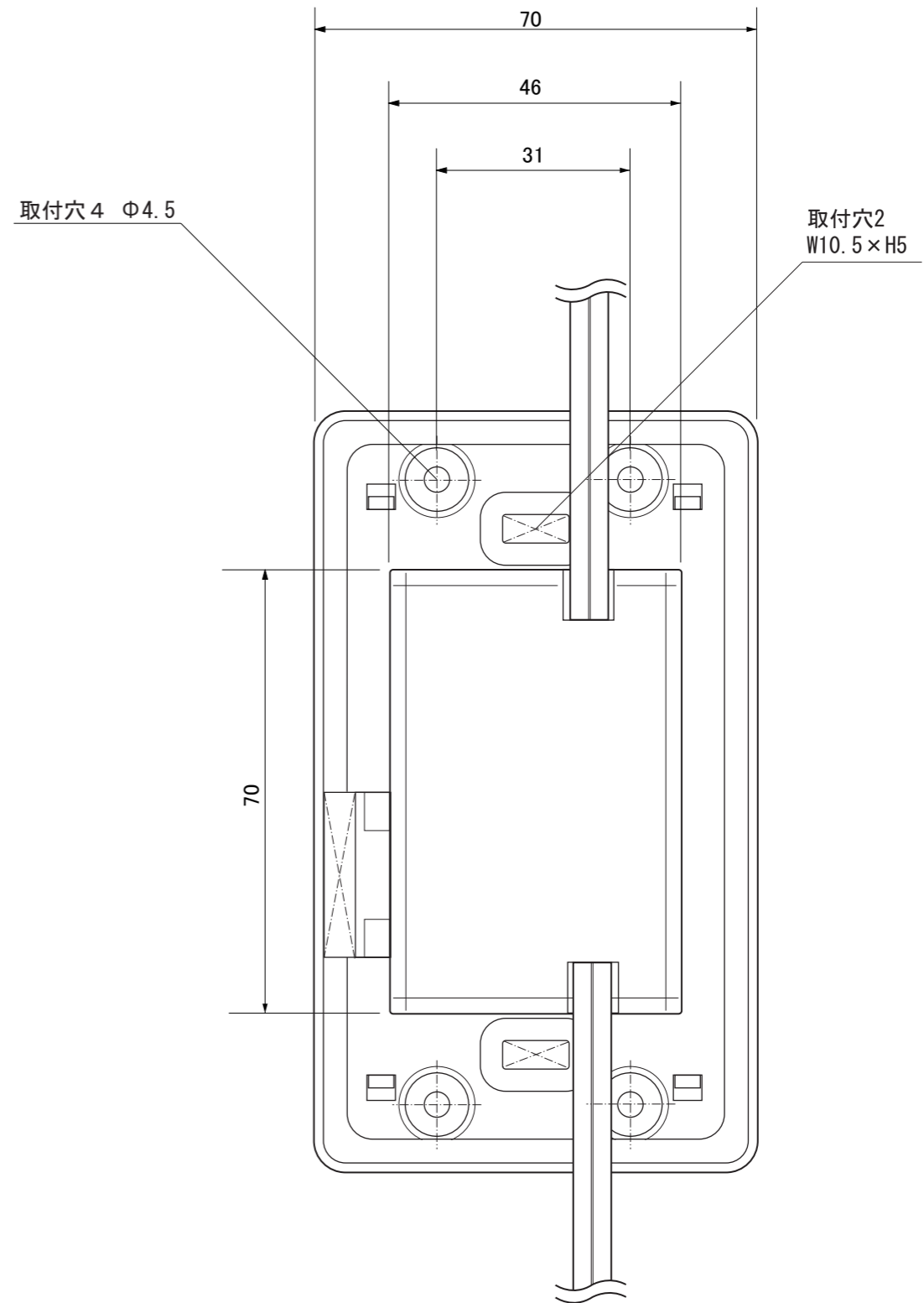
【背面図】
