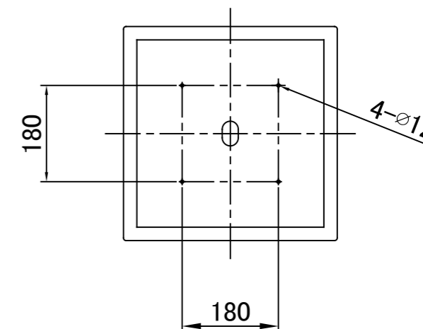
A-1 ■ 取付寸法図
