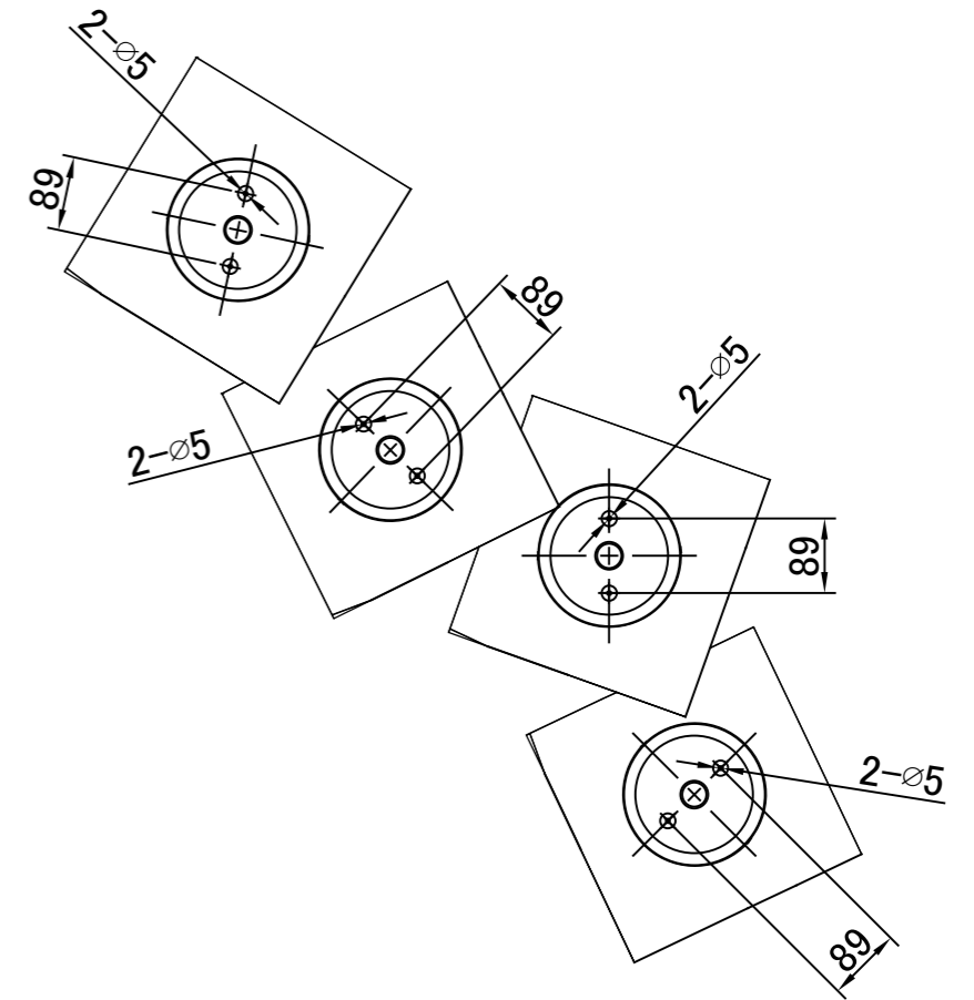
A-1 ■取付寸法図
