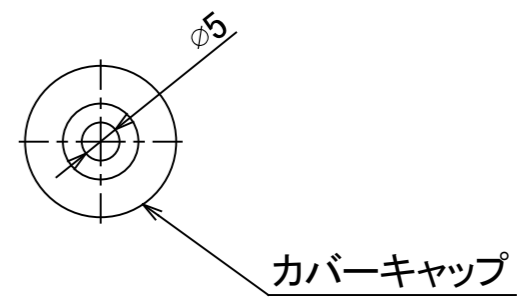
A-1 ■取付寸法図
