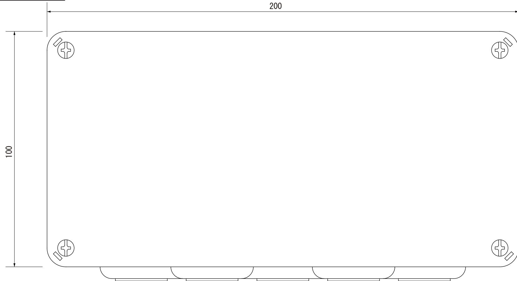
【正面図】
