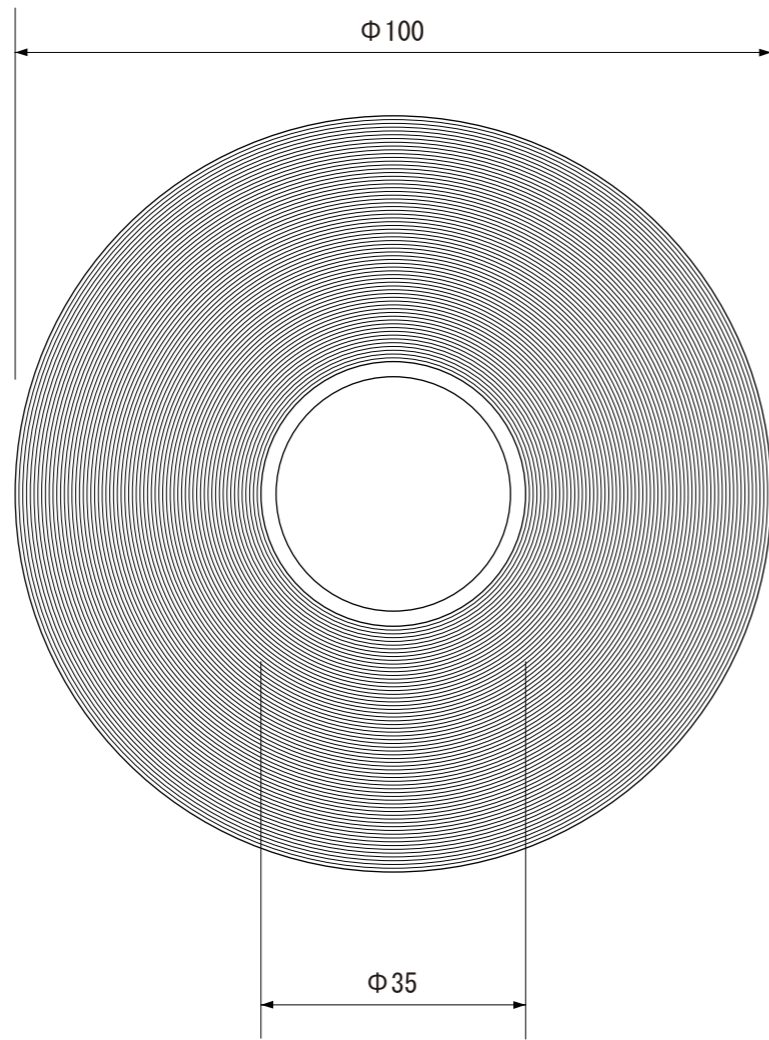
【正面図】
