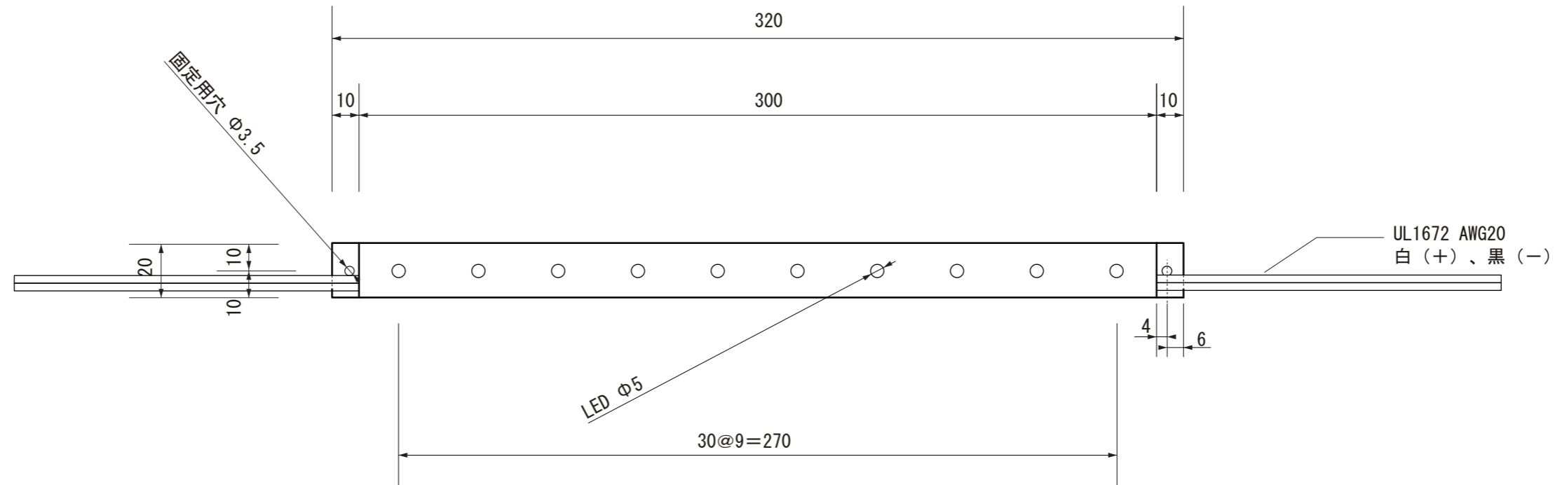
【上面図】
