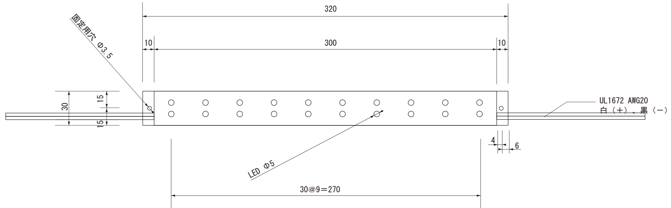
【上面図】
