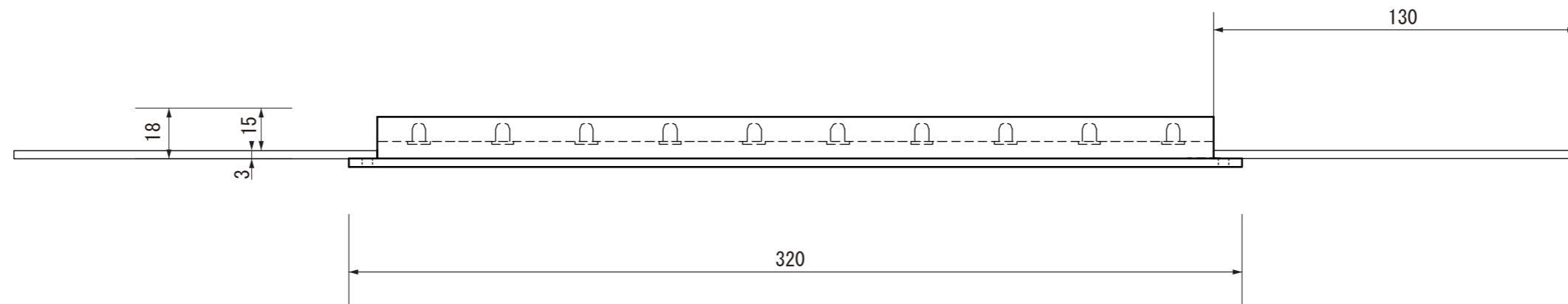
【正面図】
