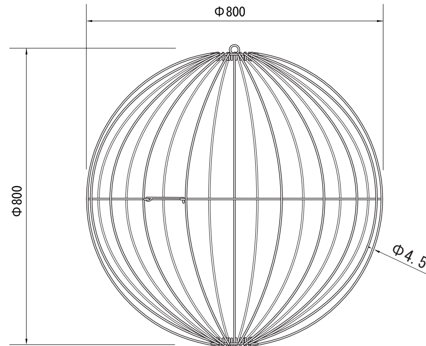
【正面図】
