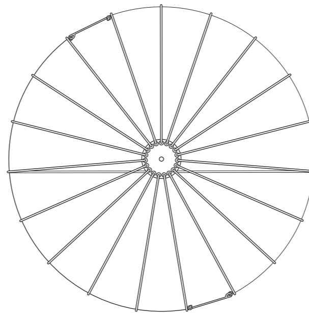
【底面図】
