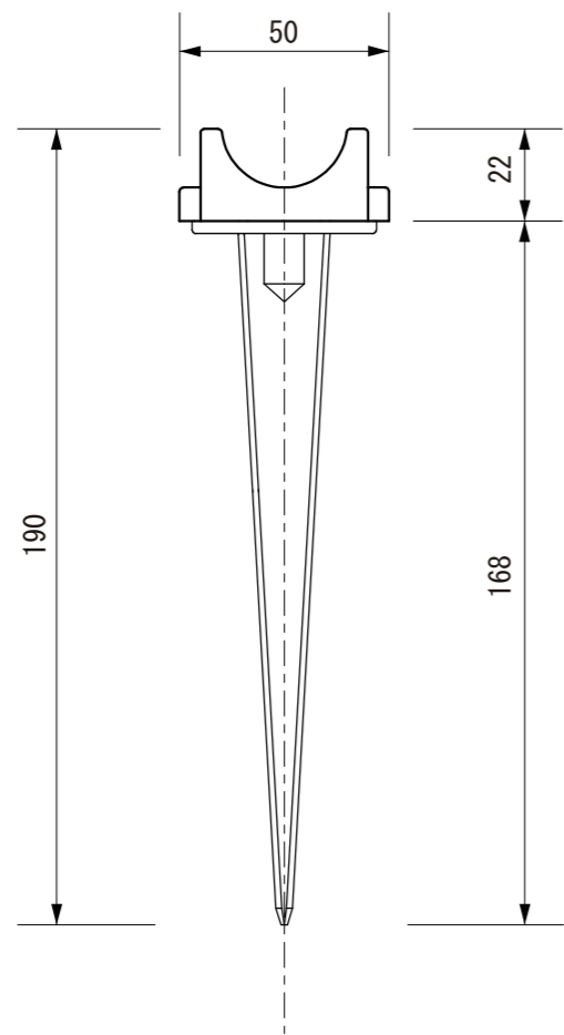
【正面図】
