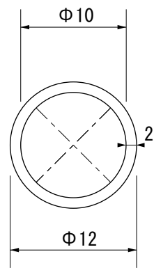
【正面図】
