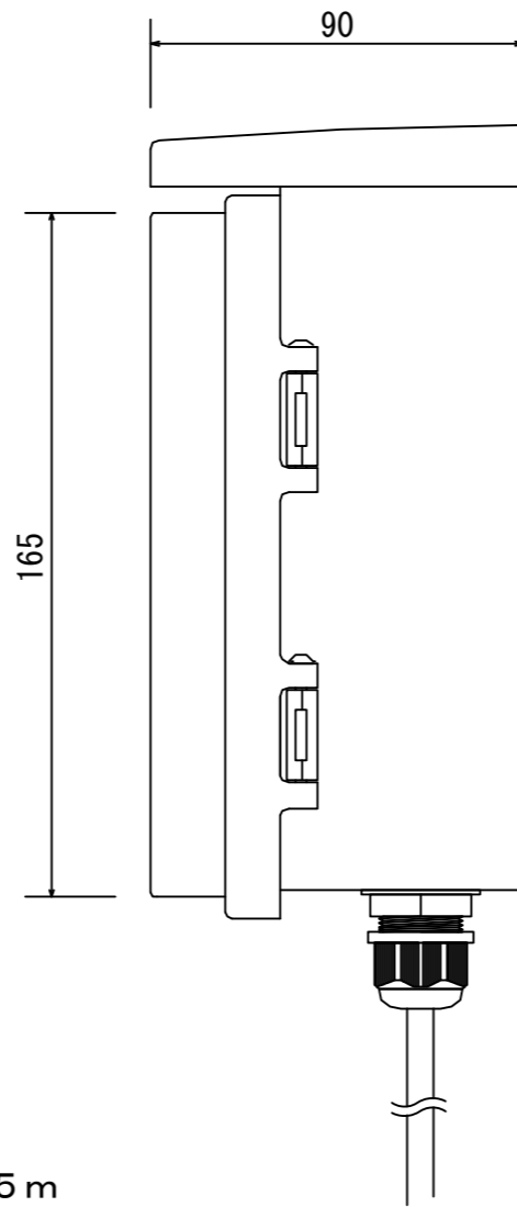
【側面図】
