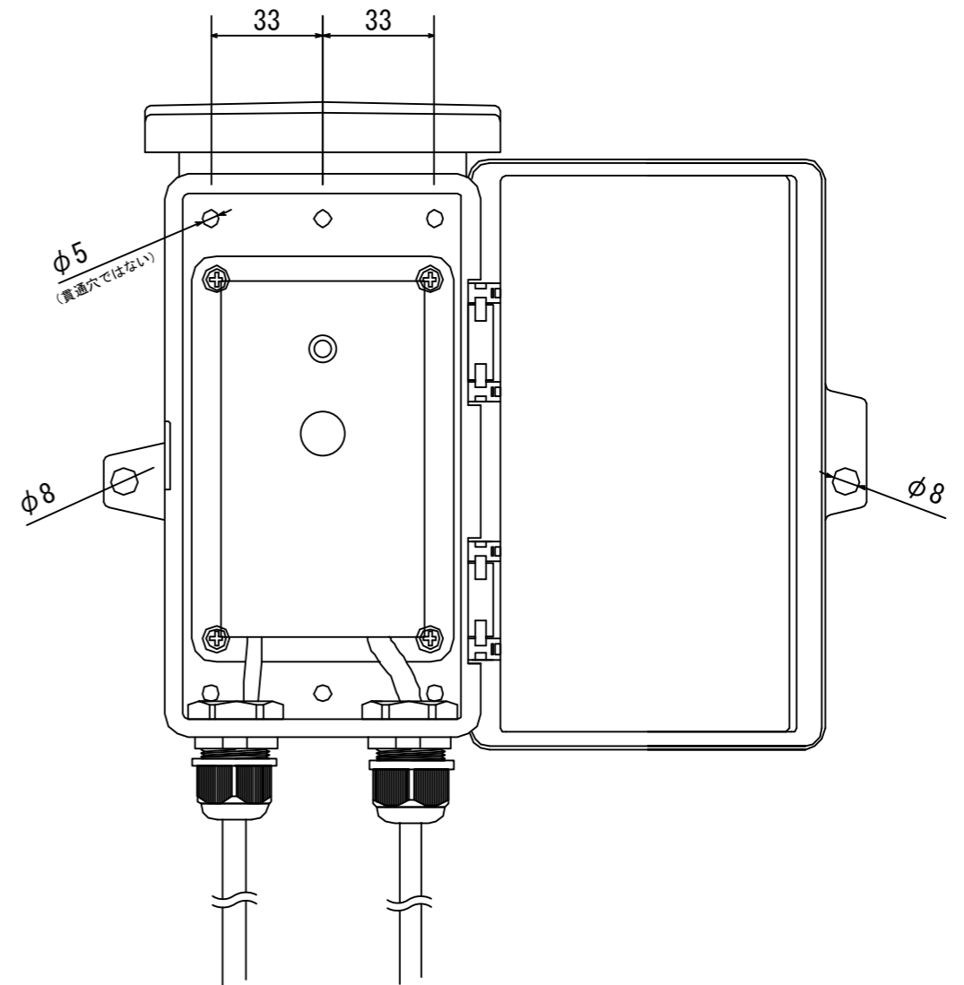
【正面図】
