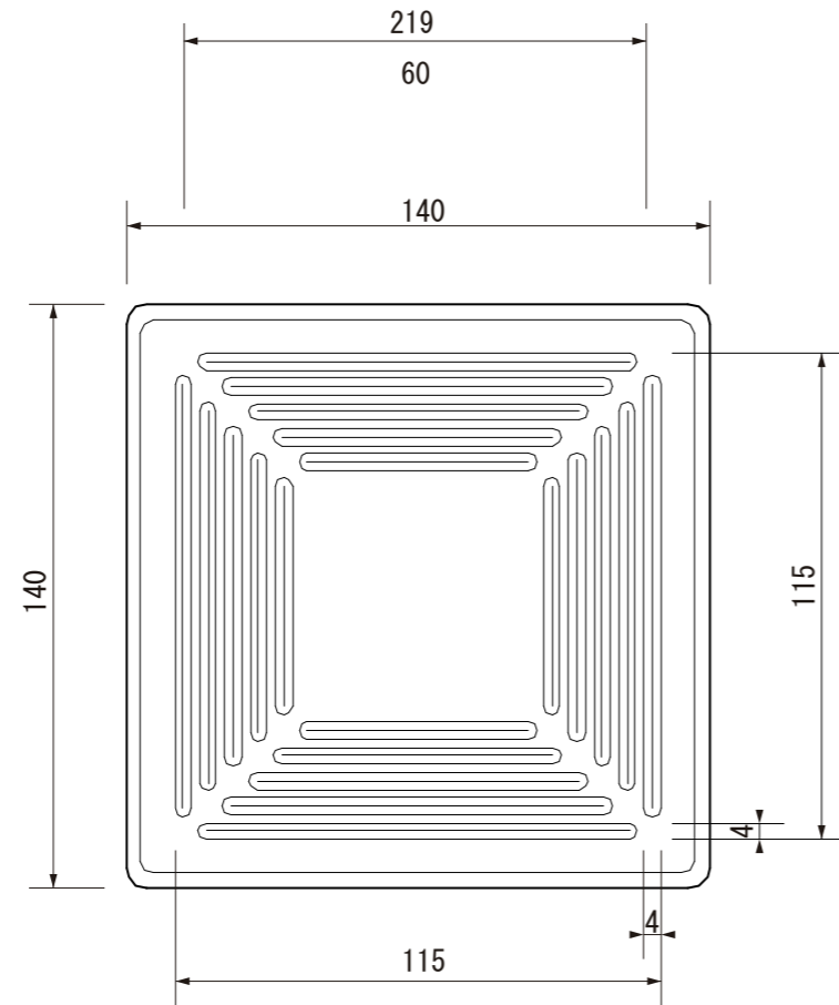
【上面図】
