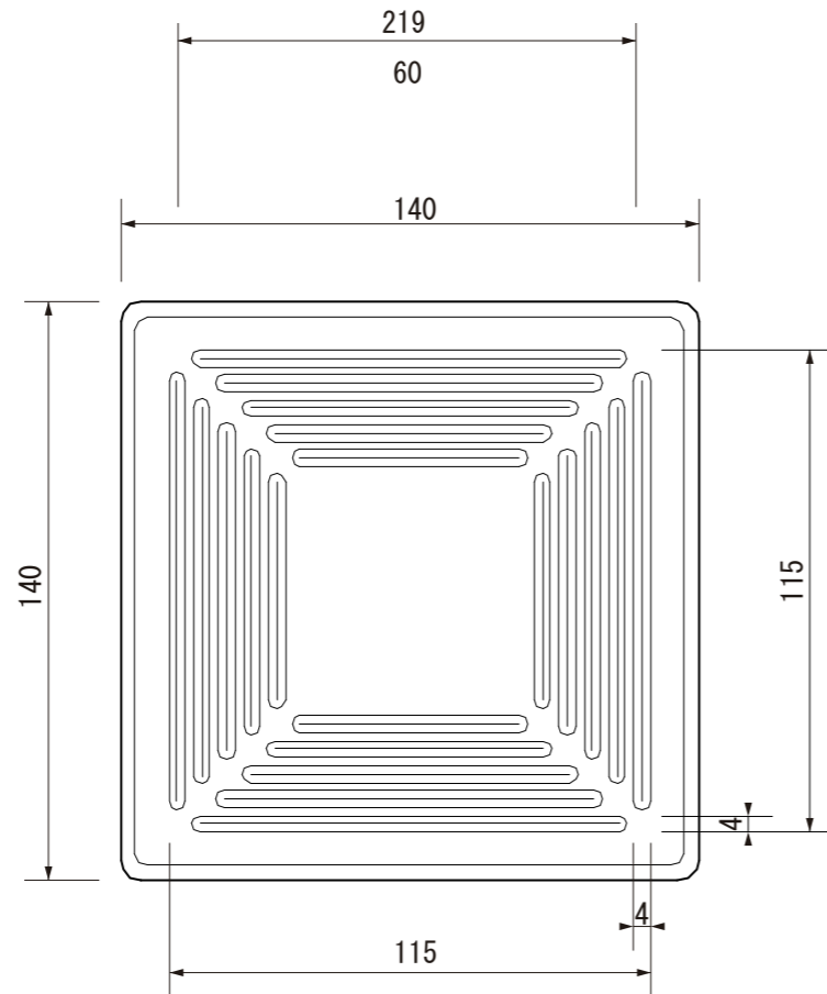
【上面図】
