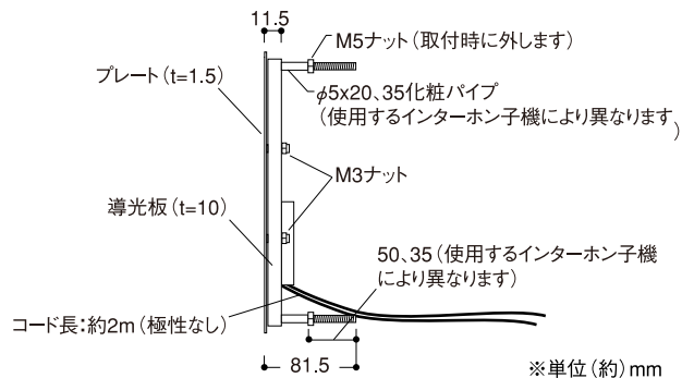
側面図 100Vタイプ
