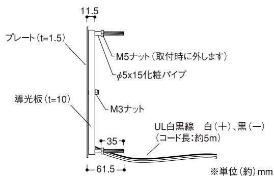
側面図 ローボルトタイプ
