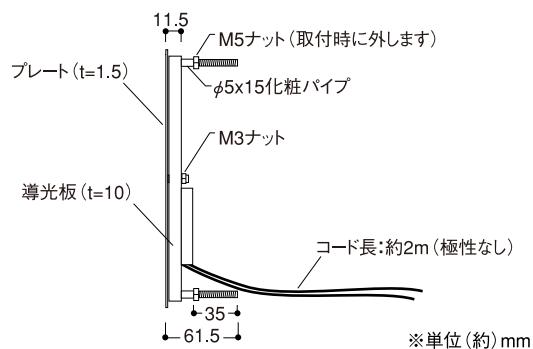
側面図 100Vタイプ
