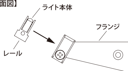
【側面図】
