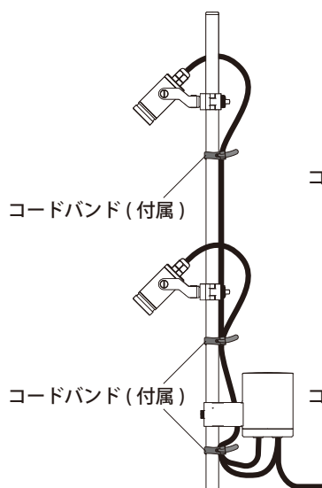
【灯具2灯の場合】
