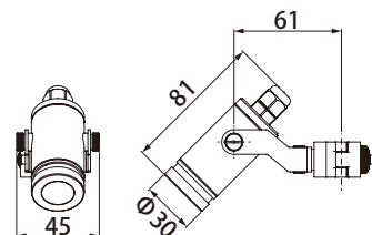
追加用灯具 HBB-D145C
