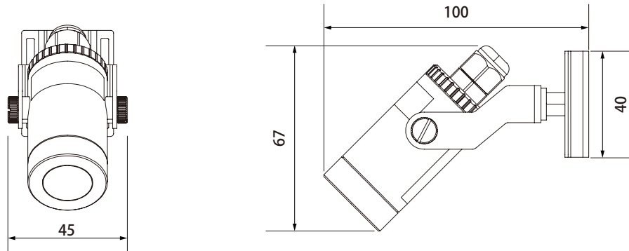
首振り45°の時
