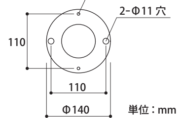
■取付面(ベースプレート) 2-Φ5穴
