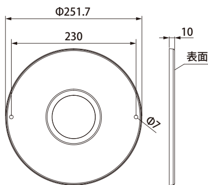
化粧パネル
