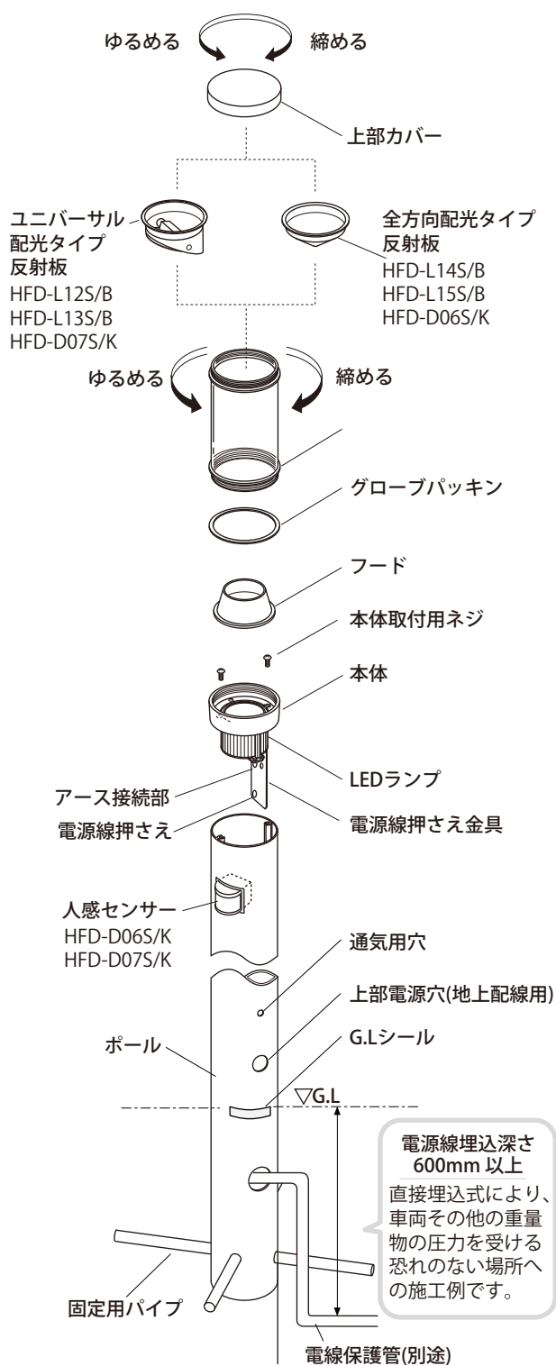
【図D】 各部の名称図
