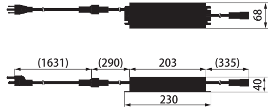
36Vトランス 200W MKA-T07X
