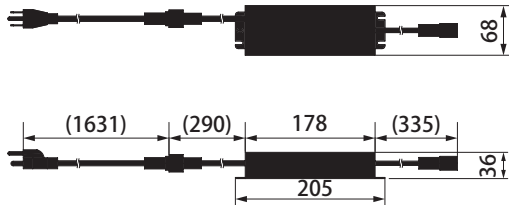
36Vトランス 90W MKA-T06X
